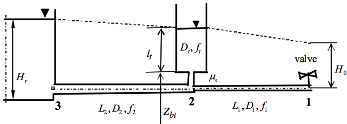
Figura 3 - Sistema hidráulico a ser otimizado. Fonte: NEAGOE & POPA, 2013.
