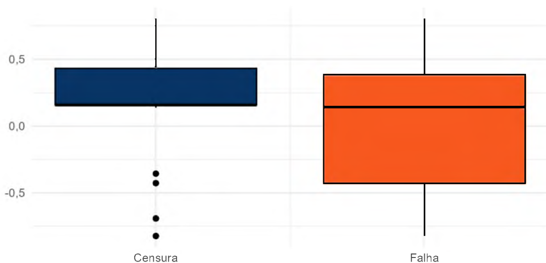
Figura 23: Boxplots da Ideologia do Governador pelo Status de adoção das políticas.
