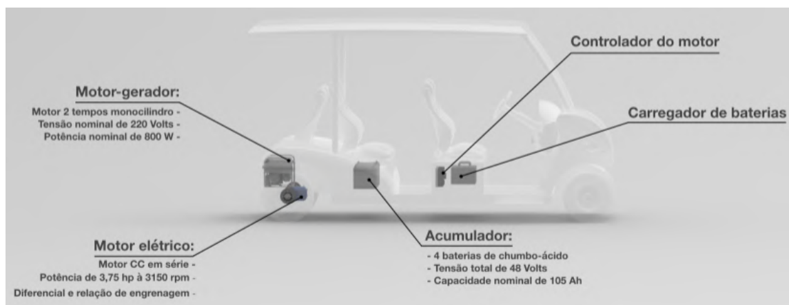
Figura 23 – Posição dos componentes do carro de golfe híbrido da UnB-FGA, autoria própria.
