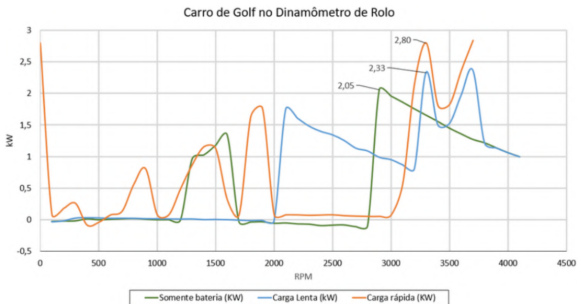
Figura 28 – Curvas de potência pela rotação do carro de golfe híbrido da UnB, retirado de: OLIVEIRA .
