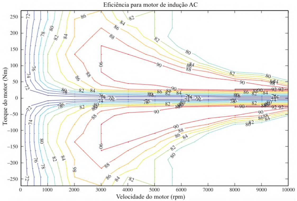
Figura 5 – Mapa de eficiência para motor de indução, adaptado de: LIU .
