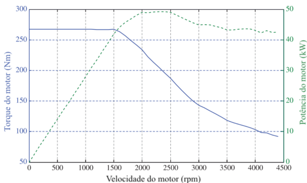
Figura 7 – Gráfico torque/potência para um motor BLDC teórico, adaptado de: LIU.
