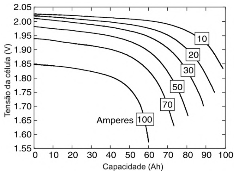
Figura 12 – Descarga de uma bateria de chumbo-ácido com relação a capacidade nominal, adaptado de: EMADI ; GAO ; EHSANI .
