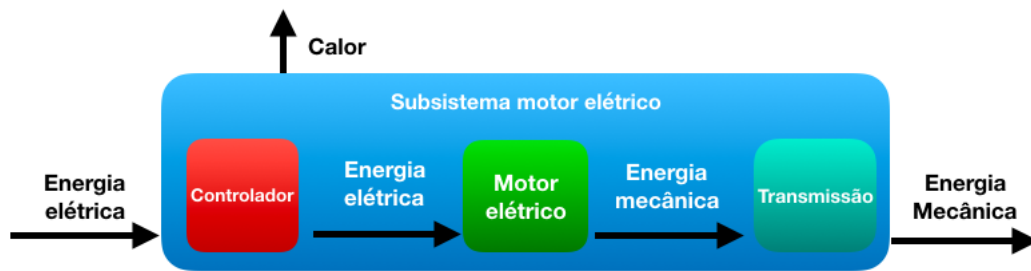
Figura 29 – Diagrama de blocos para o subsistema motor elétrico, autoria própria.
