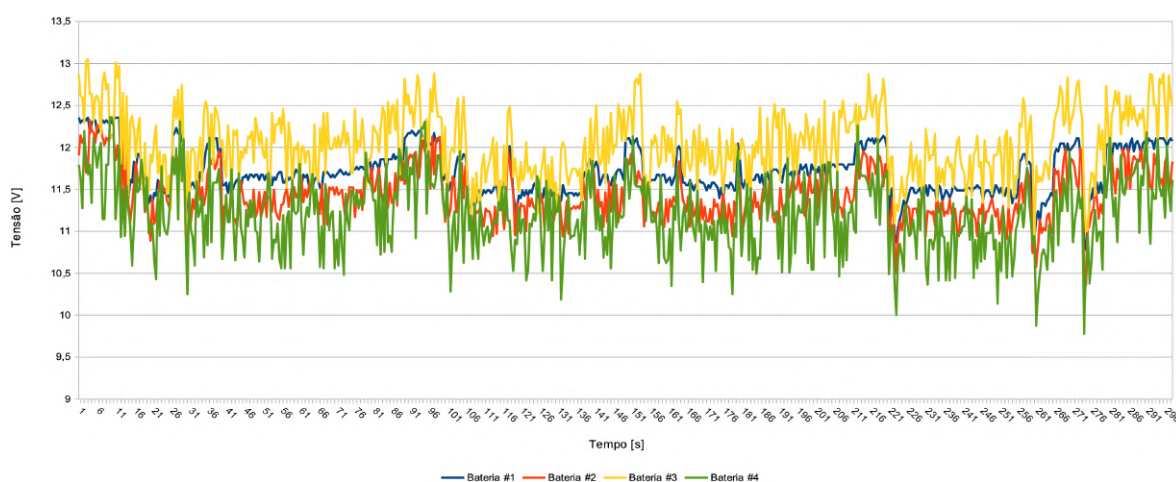
Figura 69 – Dados de tensão das baterias no ensaio 1.
