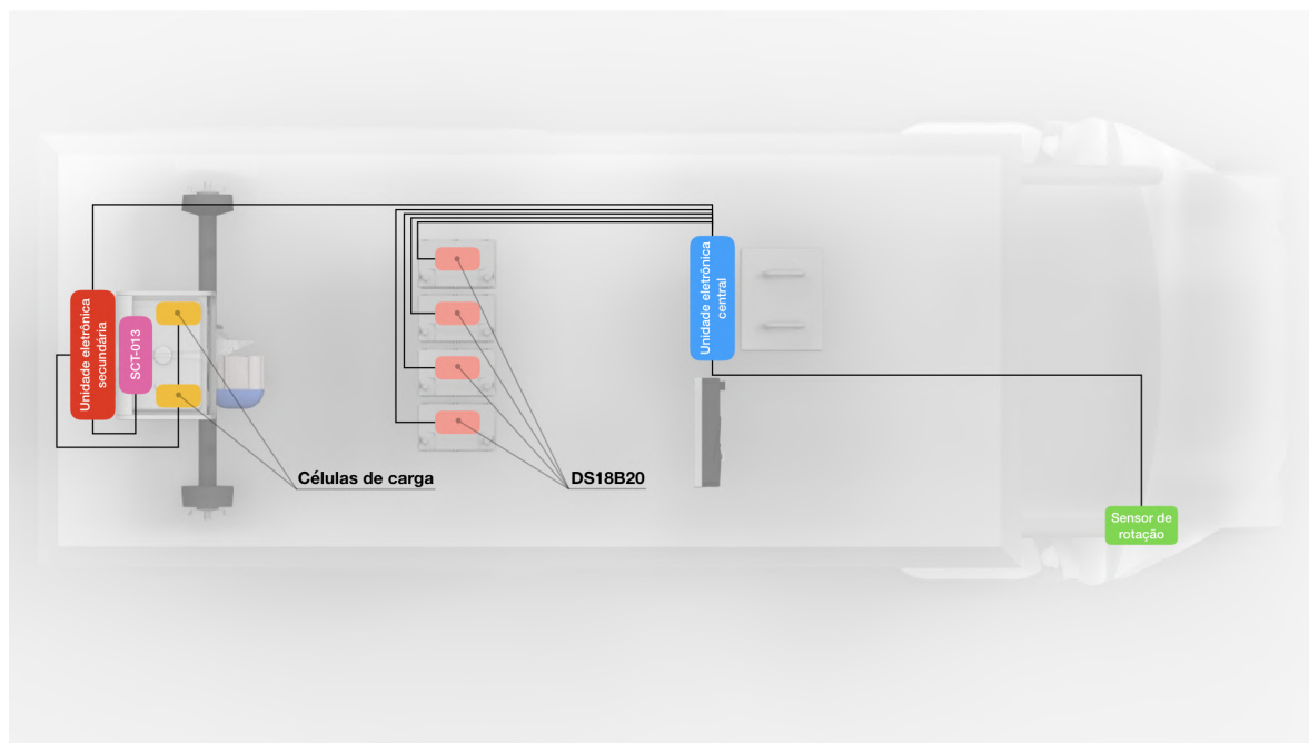
Figura 60 – Local de instalação das unidades e componentes do sistema COLUMBUS.
