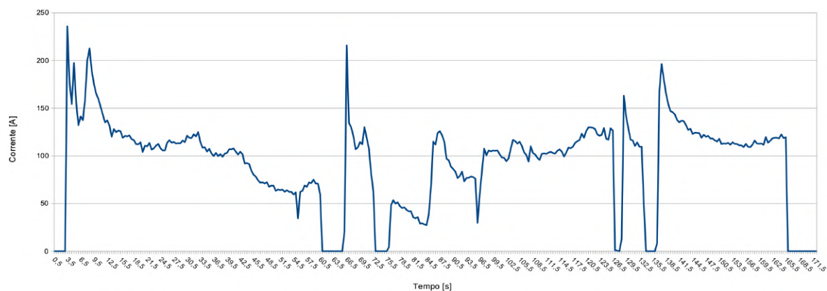
Figura 77 – Dados de corrente elétrica no ensaio 3.
