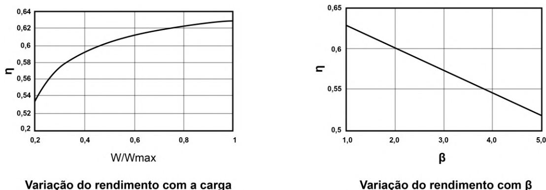
Figura 1 – Rendimento com relação à carga e \beta , retirado de: MARTINS
