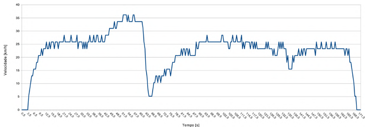
Figura 78 – Dados de velocidade do veículo no ensaio 3.
