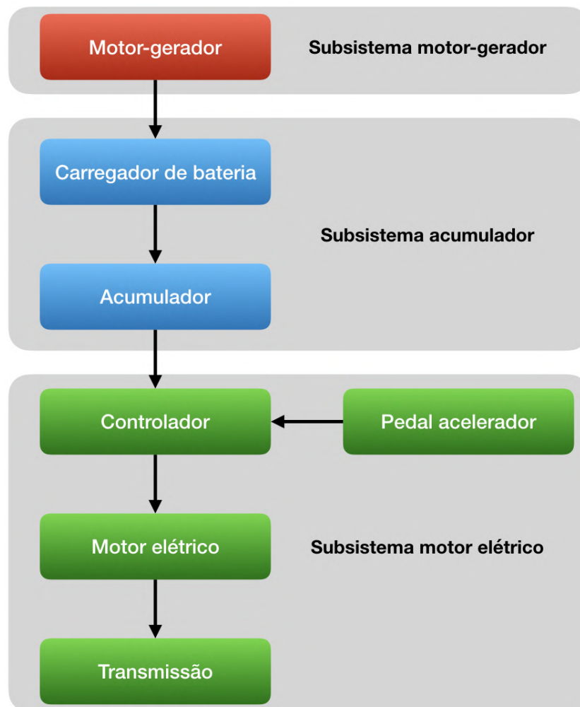
Figura 22 – Diagrama esquemático de comunicação entre componentes de um VHE em série típico, autoria própria.
