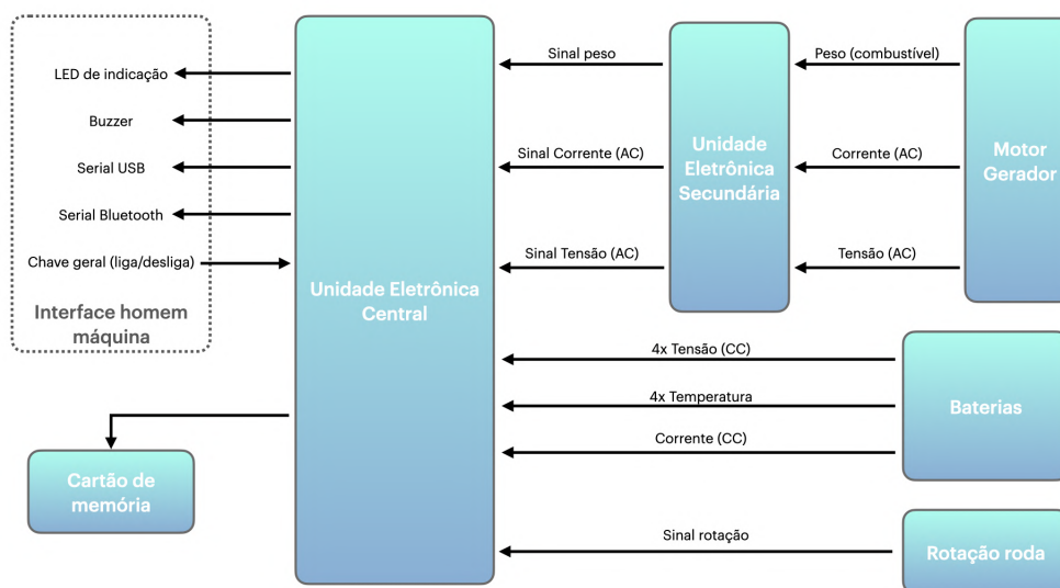
Figura 35 – Diagrama de blocos para o sistema de aquisição de dados, autoria própria.
