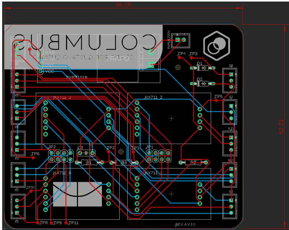
Figura 53 – Placa de circuito impresso da unidade eletrônica secundária.
