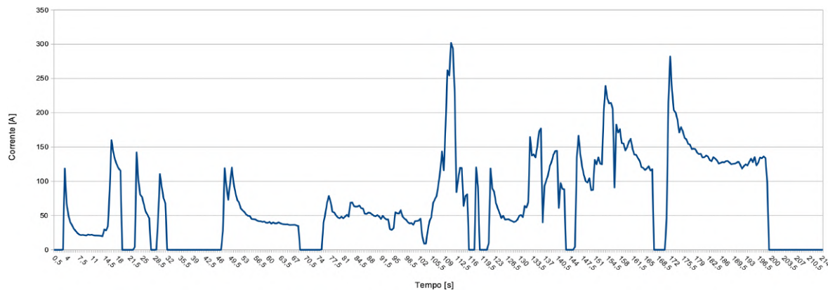
Figura 72 – Dados de corrente elétrica no ensaio 2.
