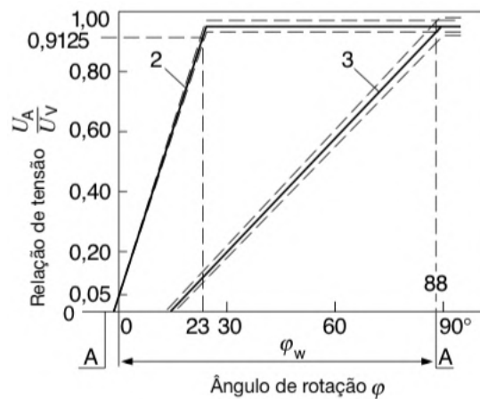
Figura 21 – Função de transferência do sensor TPS da BOSCH, adaptado de: BOSCH.
