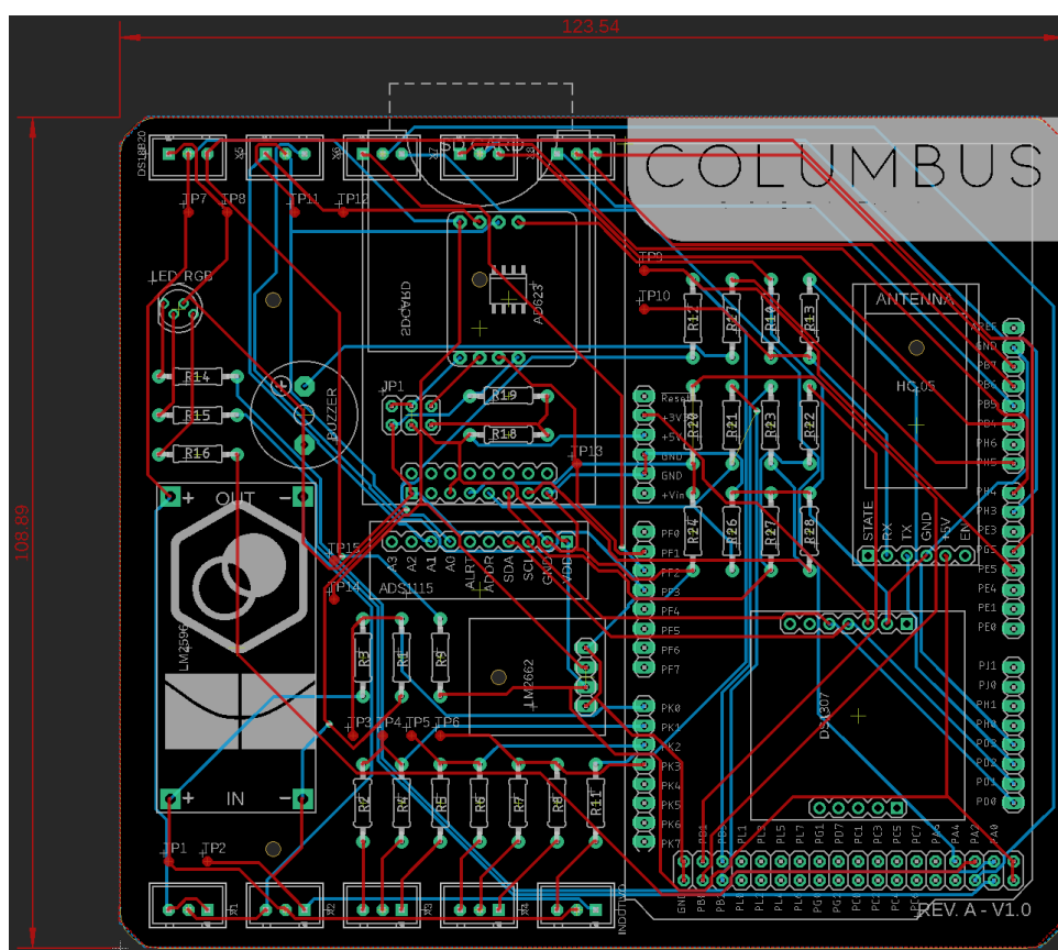
Figura 50 – Circuito da unidade central eletrônica do projeto COLUMBUS.
