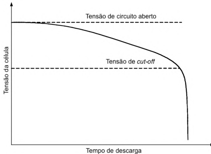
Figura 11 – Comportamento de cut-off de uma bateria típica, adaptado de: EMADI; GAO; EHSANI .
