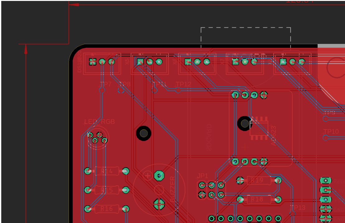
Figura 51 – Preenchimento das lacunas da PCB com o aterramento do circuito.
