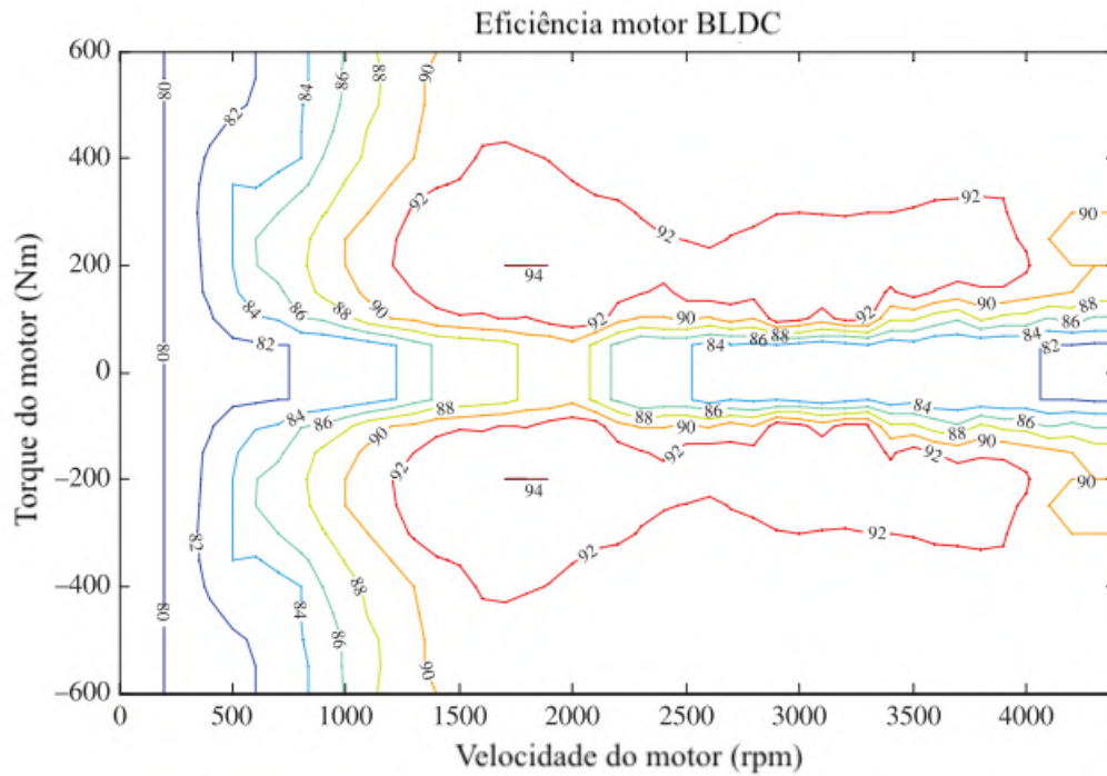
Figura 8 – Mapa de eficiência para um motor BLDC, adaptado de: LIU.
