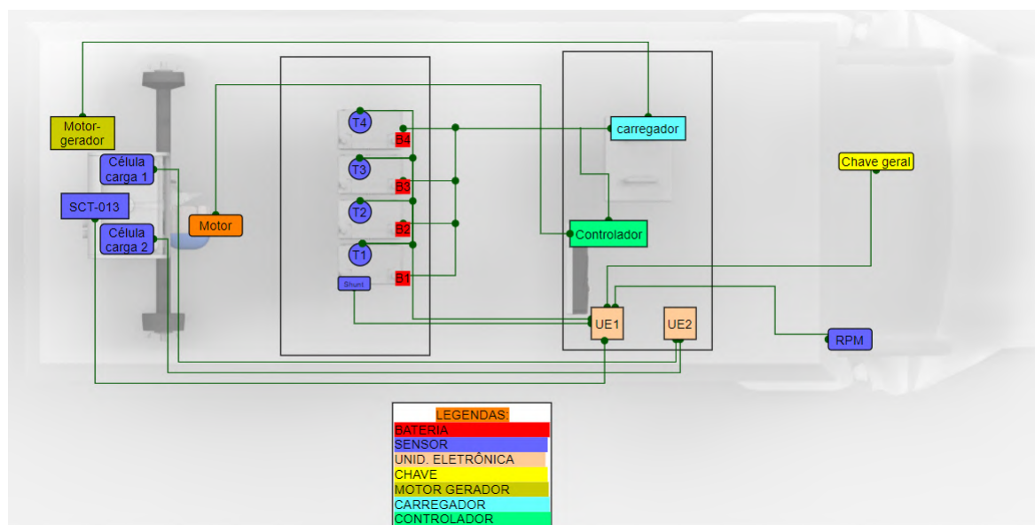
Figura 64 – Diagrama de conexões elétricas, autoria própria.
