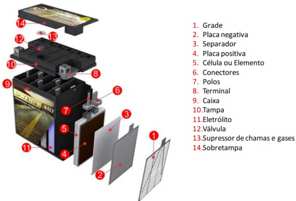
Figura 10 – Componentes de uma bateria de chumbo-ácido regulada por válvula, retirado de: CARNEIRO et al. .
