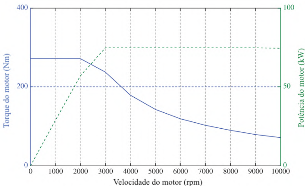
Figura 4 – Curva de torque/potência típica de um motor de indução, adaptado de: LIU
