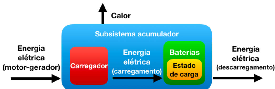
Figura 26 – Diagrama de blocos para o subsistema acumulador, autoria própria.
