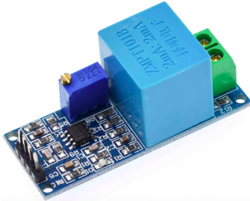
Figura 36 – Módulo ZMPT101B para medições de tensão AC até 250 V.
