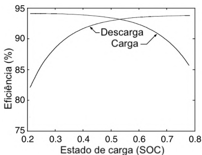
Figura 13 – Eficiência energética de uma bateria de chumbo-ácido para carga e descarga, adaptado de: EMADI ; GAO ; EHSANI .
