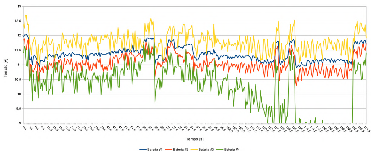
Figura 79 – Dados de tensão das baterias no ensaio 3.
