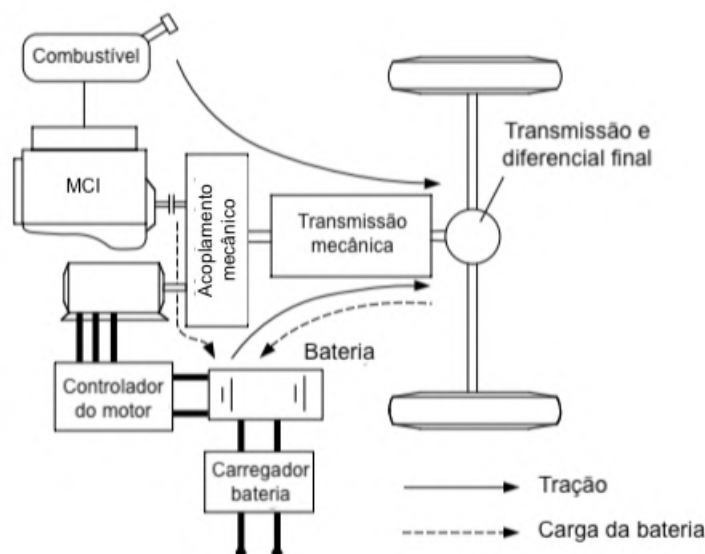
Figura 18 – Configuração de um VHE em paralelo, adaptado de: EMADI ; GAO ; EHSANI .
