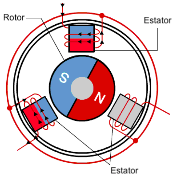
Figura 6 – Funcionamento de um motor BLDC, adaptado de: Renesas .
