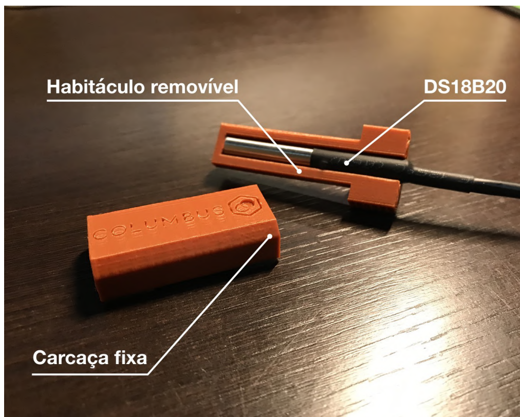
Figura 62 – Protótipo do elemento de fixação para o DS18B20.
