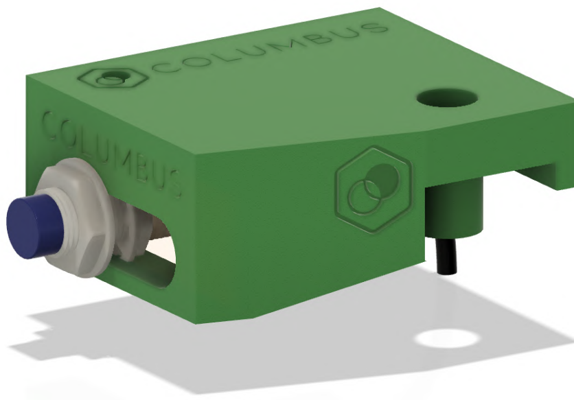
Figura 63 – Modelo CAD do suporte do sensor de relutância variável.
