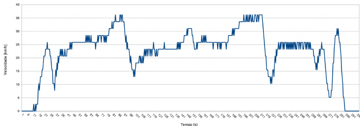
Figura 68 – Dados de velocidade do veículo no ensaio 1.
