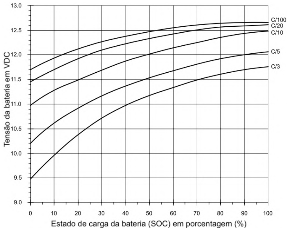
Figura 14 – Estado de carga relacionado a tensão de baterias 12 V de chumbo-ácido durante descarga, adaptado de: PEREZ.
