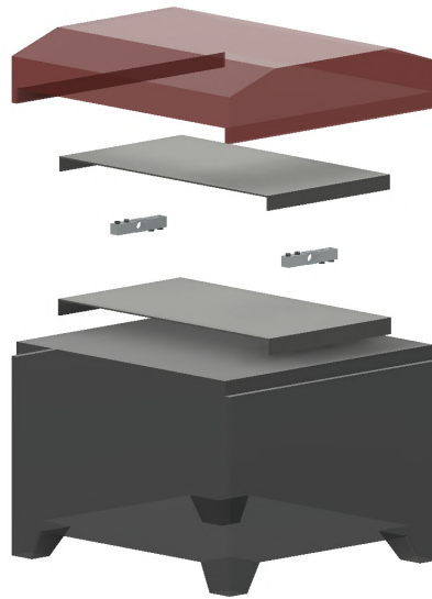
Figura 61 – Vista explodida da posição das células de carga sobre o tanque de combustível.
