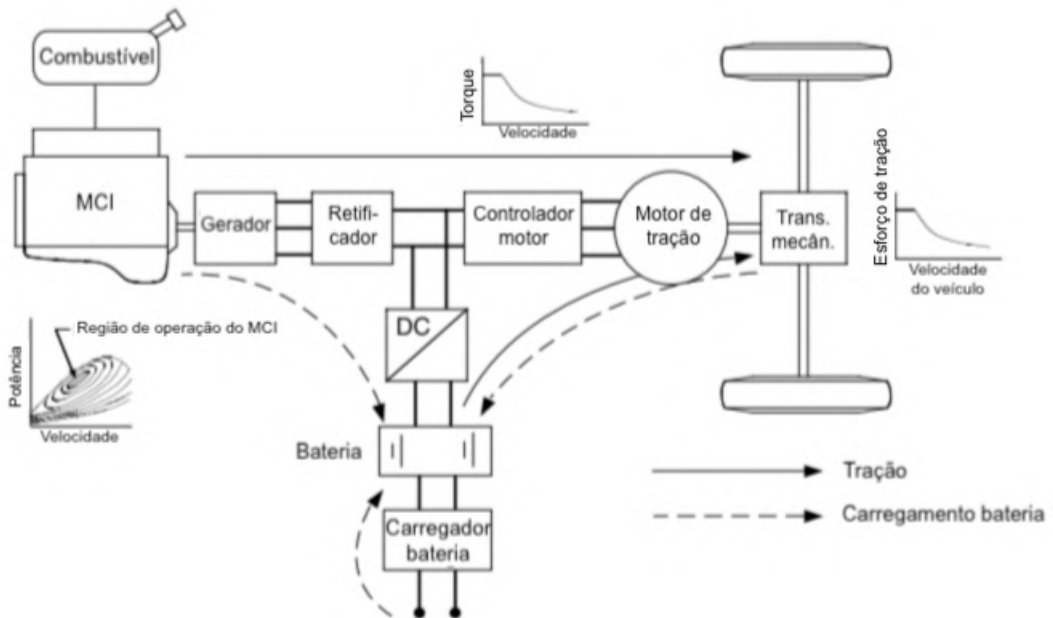
Figura 17 – Arquitetura de um VHE em série, adaptado de: EMADI; GAO; EHSANI.
