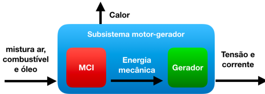
Figura 25 – Diagrama de blocos para o subsistema motor-gerador, autoria própria.
