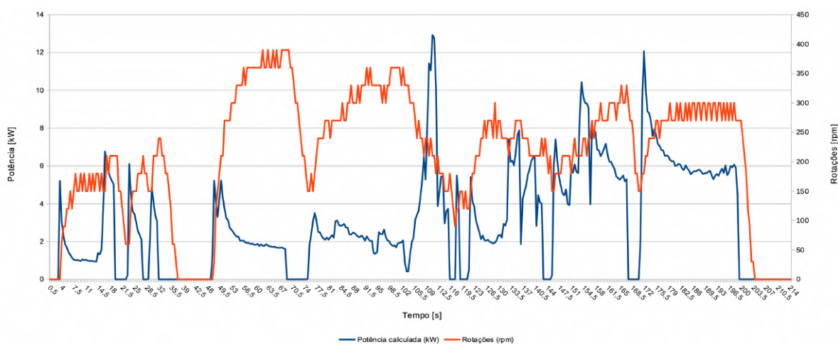
Figura 71 – Dados de potência calculada e rotação da roda no ensaio 2.
