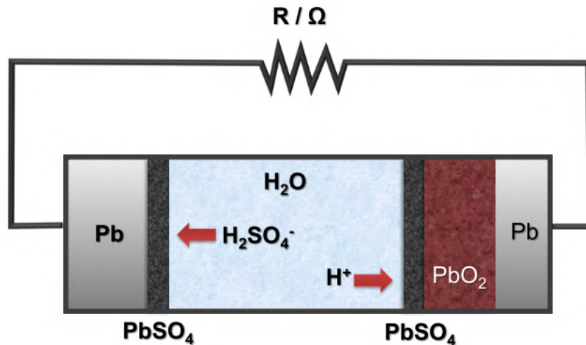
Figura 9 – Processo esquemático do descarregamento de uma bateria de chumbo-ácido, retirado de: CARNEIRO et al. .
