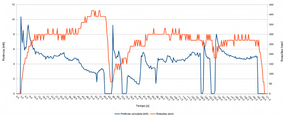
Figura 76 – Dados de potência calculada e rotação da roda no ensaio 3.
