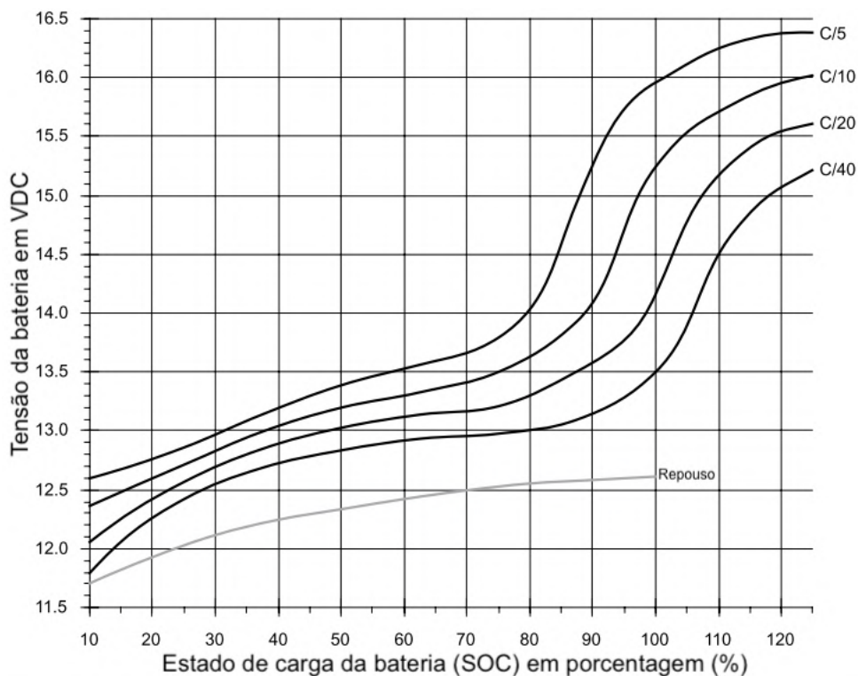
Figura 15 – Estado de carga relacionado a tensão de baterias 12 V de chumbo-ácido durante recarga, adaptado de: PEREZ.
