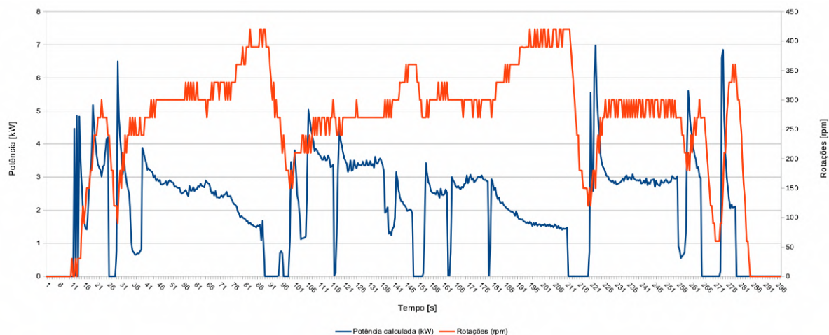
Figura 66 – Dados de potência calculada e rotação da roda no ensaio 1.
