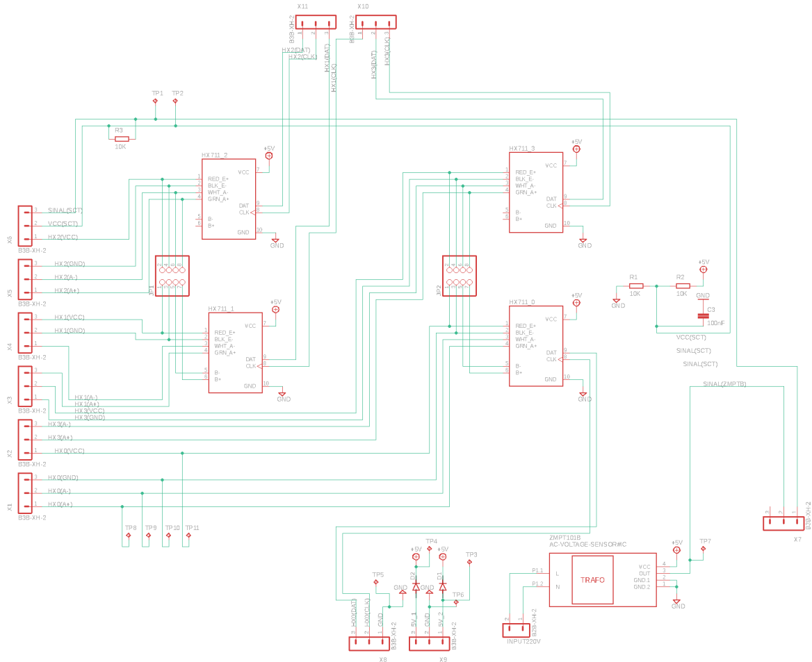
Figura 52 – Esquemático da unidade eletrônica secundária.
