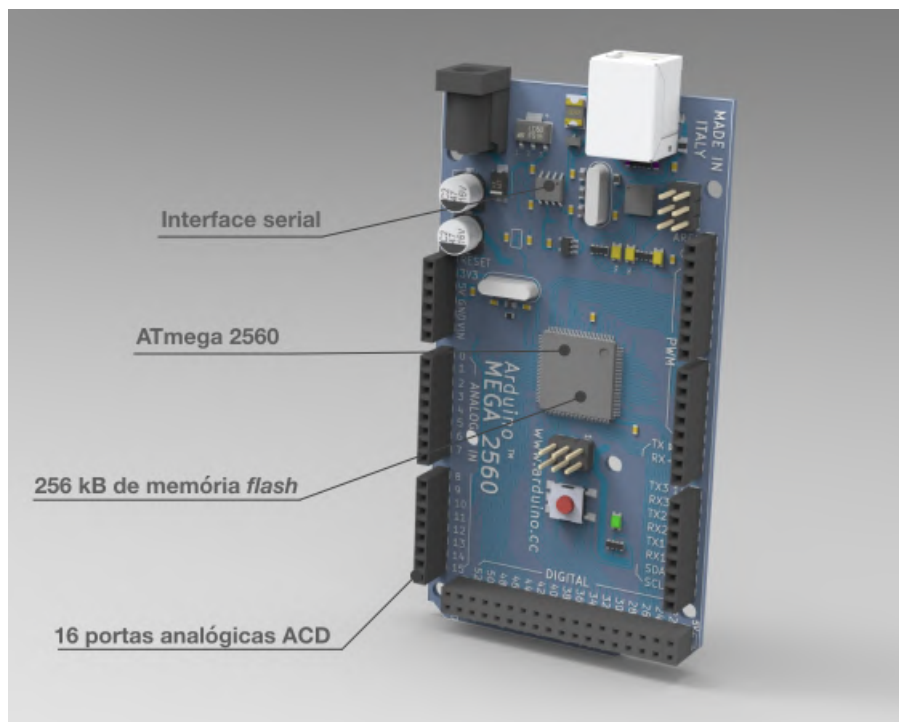
Figura 34 – Funções do Arduino Mega e ATmega2560, autoria própria.
