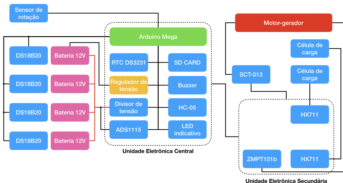
Figura 42 – Esquema das unidades eletrônicas do projeto COLUMBUS, autoria própria.
