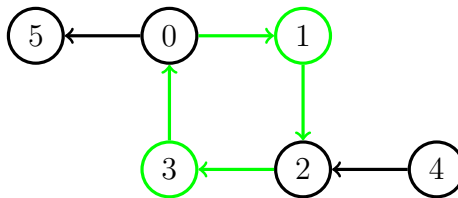
Figura 5 – Exemplo de nós fortemente conectados em verde
