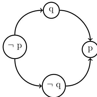
Figura 11 – Grafo FNI da Equação 2.15
