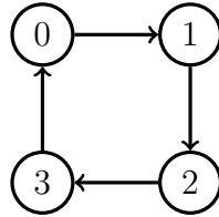
Figura 4 – Exemplo de um grafo fortemente conectado
