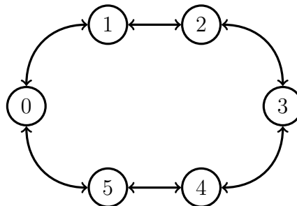
Figura 2 – Exemplo de um grafo bidirecional
