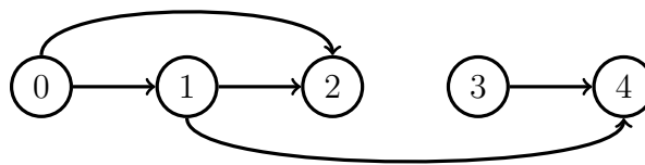
Figura 8 – Grafo da Figura 1 na ordem topológica
