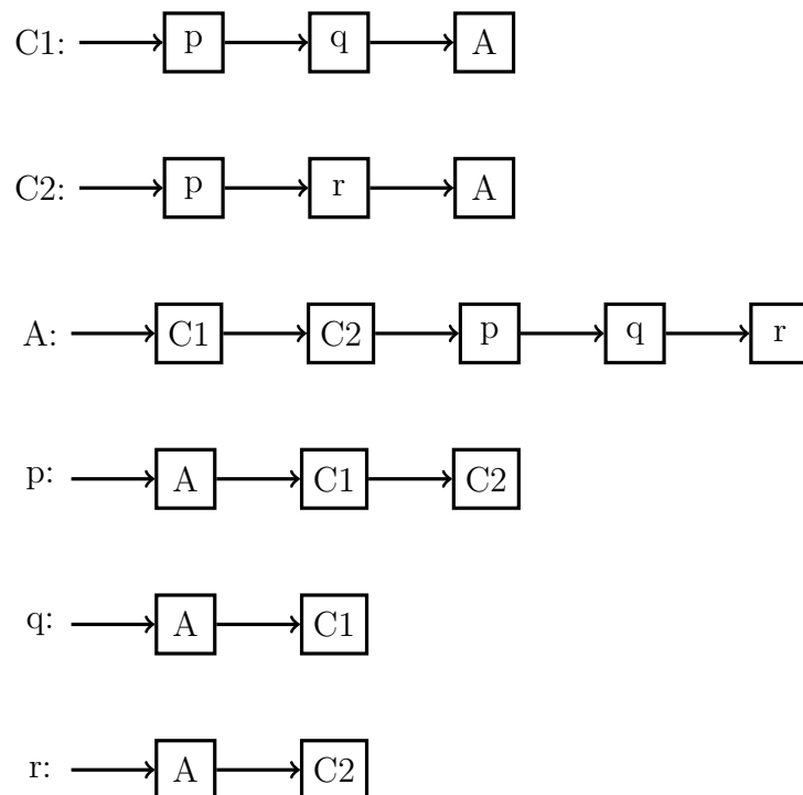
Figura 13 – Lista de adjacências obtidas através da Equação 3.2
