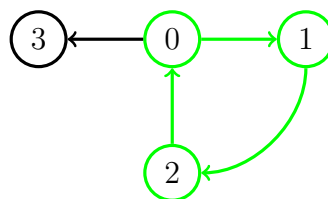
Figura 6 – Exemplo de CFC em verde
