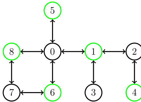
Figura 7 – Exemplo de CIM representado pelos nós em verde
