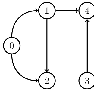
Figura 1 – Exemplo de um grafo unidirecional
