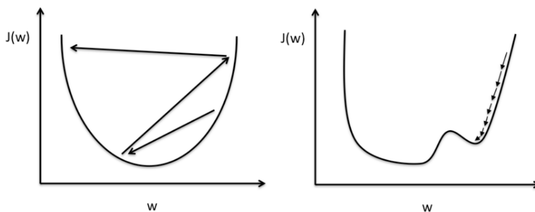
Figura 2.9: Efeitos da taxa de aprendizado na minimização da função de custo. O gráfico da esquerda mostra uma divergência no treinamento causado por uma taxa de aprendizado alta, e o gráfico da direita mostra a perda de um mínimo global por causa do uso de uma taxa de aprendizado muito baixa. Reproduzida de [8].
