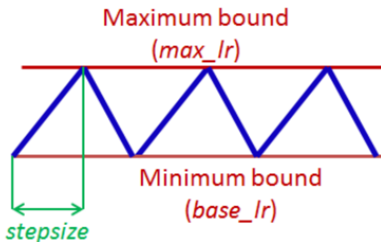
Figura 2.10: A taxa de aprendizado triangular. Reproduzida de [9]. ©2017 IEEE.
