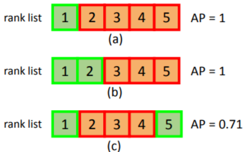
Figura 4.5: Comparação entre as métricas AP e CMC. Para esses três exemplos e utilizando uma abordagem de top-5 predições, tem-se que a métrica CMC vale 1 para todos, enquanto a métrica AP tem resultados que variados. Reproduzida de [15]. ©2015 IEEE.
