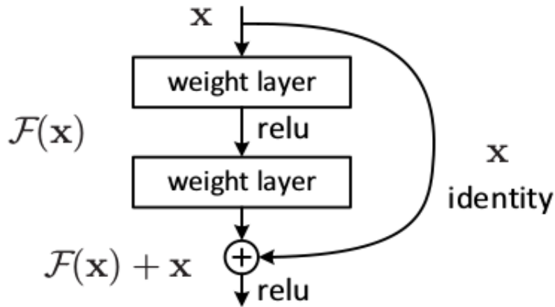
Figura 2.6: Funcionamento de um bloco residual. Reproduzida de [5]. ©2016 IEEE
