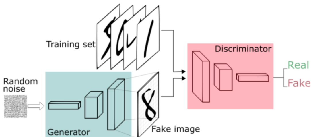
Figura 2.12: Fluxo de dados nas redes geradora e discriminativa de uma GAN. Reproduzida de [11].
