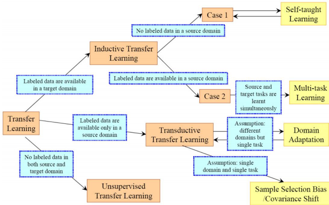
Figura 2.11: Classificação dos tipos de transferência de aprendizado definidos por Pan e Yang. Reproduzida de [10]. ©2010 IEEE.
