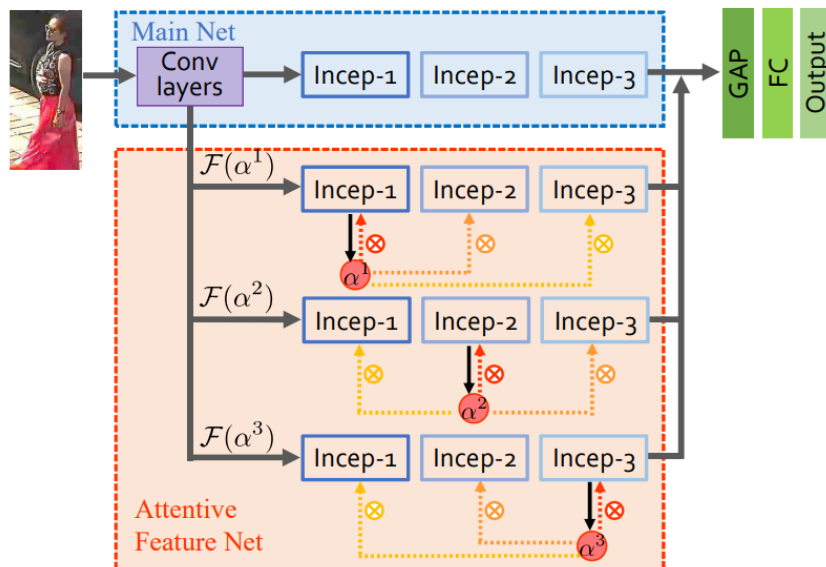
Figura 5.1: Rede HP-net responsável pelo melhor resultado já publicado na base de dados CUHK03 . Reproduzida de [21]. ©2017 IEEE.
