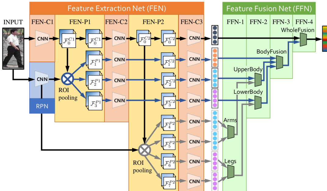
Figura 5.2: Rede Spindle responsável pelo melhor resultado já publicado na base de dados Viper . Reproduzida de [22]. ©2017 IEEE.
