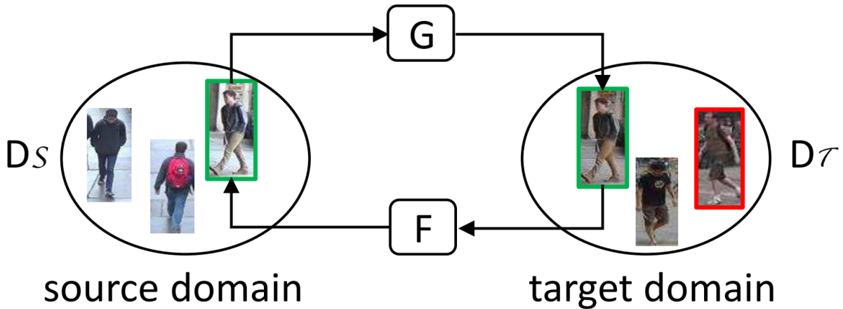
Figura 4.4: Exemplo do funcionamento das funções geradoras F e G aprendidas por uma GAN cíclica. Onde, D_\tau = d_{alvo} (domínio alvo) e D_s = D_{fonte} (domínio fonte). Reproduzida de [20]. ©2018 IEEE.
