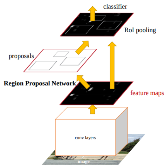
Figura 3.4: Exemplo do funcionamento de uma rede faster R-CNN , onde os atributos da rede base convolucional são combinados com a RPN para encontrar regiões interessantes na imagem e classificar essas regiões de acordo com o objeto existente nelas. Reproduzida de [17]. ©2016 IEEE.
