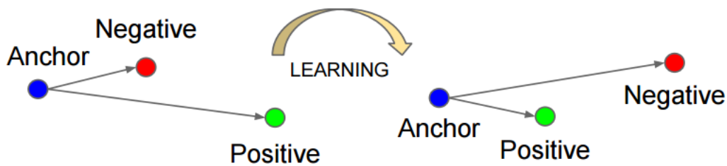
Figura 2.8: Durante o treinamento, a função de custo triplet faz com que a distância entre a imagem de treinamento ( anchor ) diminua para outras imagens da mesma pessoa e aumente para imagens de outras pessoas. Reproduzida de [7]. ©IEEE 2015.
