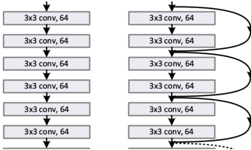
Figura 2.5: Diferença entre redes neurais simples e redes neurais que utilizam blocos residuais. A imagem da esquerda mostra os blocos simples de convolução que eram utilizados antes das arquiteturas residuais, já a imagem da direita mostra como funcionam as redes com blocos residuais. Reproduzida de [5]. ©2016 IEEE.
