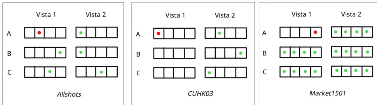
Figura 4.6: Exemplos dos tipos de comparação utilizados. Onde, A, B e C representam pessoas distintas, cada pessoa tem imagens em duas vistas e cada divisão do retângulo representa uma imagem. A divisão com um ponto vermelho representa a imagem a ser comparada e as divisões com pontos em verde representam as imagens que fazem parte do universo de comparação.
