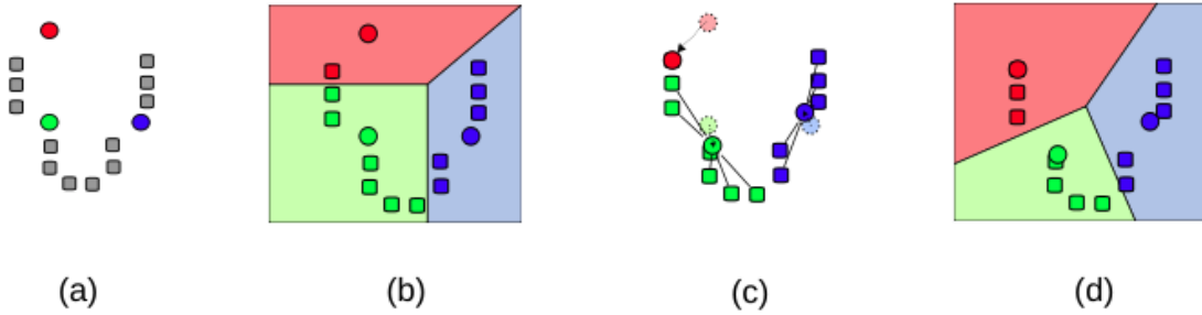
Figura 4.3: Exemplo do funcionamento do algoritmo k-means . (a) Inicialização inicial aleatória dos cluster . (b) Primeiro agrupamento, utilizando a inicialização aleatória. (c) Correção da posição dos clusters utilizando os centroides dos grupos. (d) Novo agrupamento a partir da correção da posição dos clusters . As etapas (c) e (d) são repetidas até atingir convergência ou um número máximo, pré-determinado de iterações. Reproduzida de [19].
