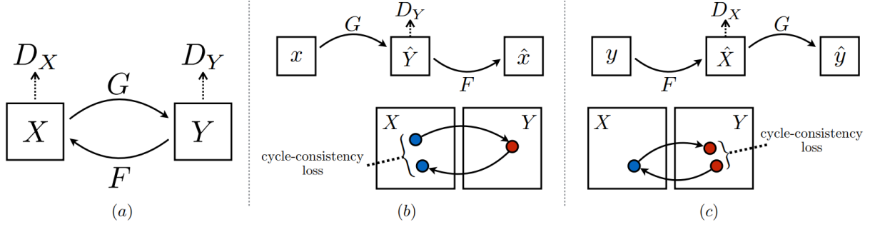
Figura 2.14: Descrição do funcionamento do modelo da GAN cíclica. (a) Modelo da GAN cíclica com duas funções geradoras G e F e duas funções discriminativas D_X e D_{X^a} , onde D_X aprende a distinguir entre imagens de X e de F(Y) e D_Y aprende a distinguir entre imagens de Y e de G(X) . (b) Exemplo do efeito do erro cíclico para aproximar F(G(X)) \approx X . (c) Exemplo do efeito do erro cíclico para aproximar F(F(Y)) \approx Y . Reproduzida de [13]. ©2017 IEEE.
