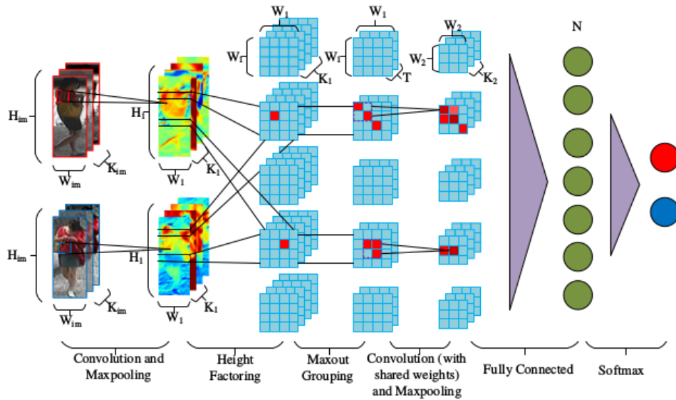
Figura 2.4: Arquitetura proposta por Li e Zhao [2]. A primeira camada combina uma convolução com uma operação de max pooling para extrair atributos robustos ao desalinhamento, enquanto a segunda camada cria uma matriz de deslocamento que indica como alinhar as partes do corpo. A terceira camada é uma camada de ativação, já quarta camada é novamente de convolução com uma operação de max pooling . A quinta camada é formada por uma operação que conecta todos os atributos da camada anterior para compensar o peso baixo que foi dado na análise do par de imagens em conjunto. Por fim, a última camada utiliza uma ativação softmax para traduzir o resultado final em uma probabilidade. Reproduzida de [2]. ©2014 IEEE.
