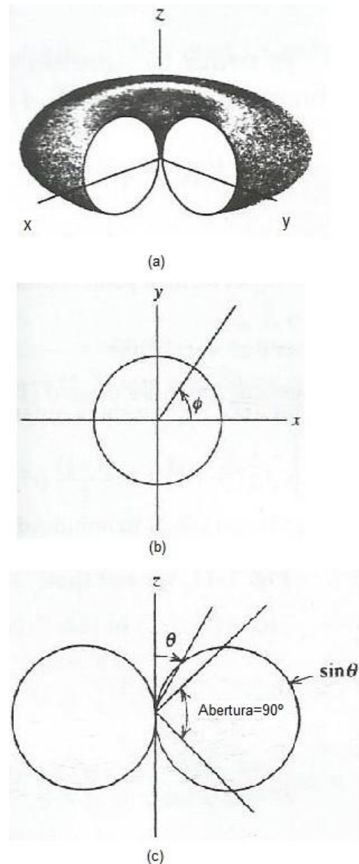
Fig.2 – Irradiação de um dipolo ideal. (a) Visão tridimensional. (b) Diagrama de irradiação horizontal. (c) Diagrama de irradiação vertical. Fonte: STUZMAN; THIELE, 1998 (adaptado).
