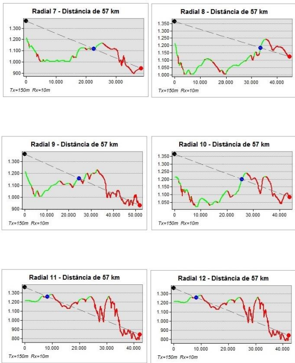
Fig.20- Contorno de 57km – Radiais de 7 a 12
