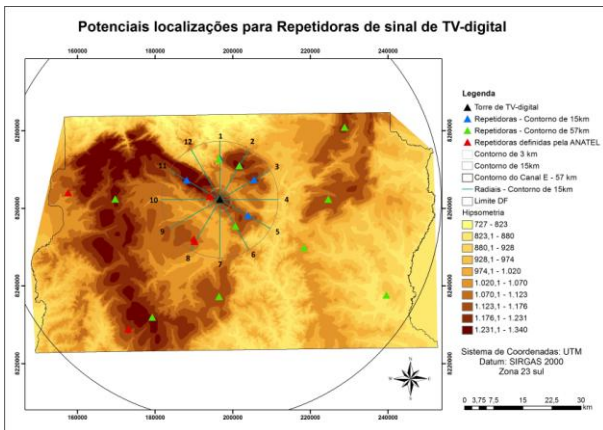
Fig. 21 – Posicionamento das repetidoras comparativamente às definidas pela Anatel
