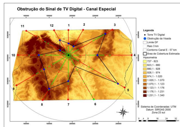
Fig.16 – Obstrução da linha de visada: contorno de 57km
