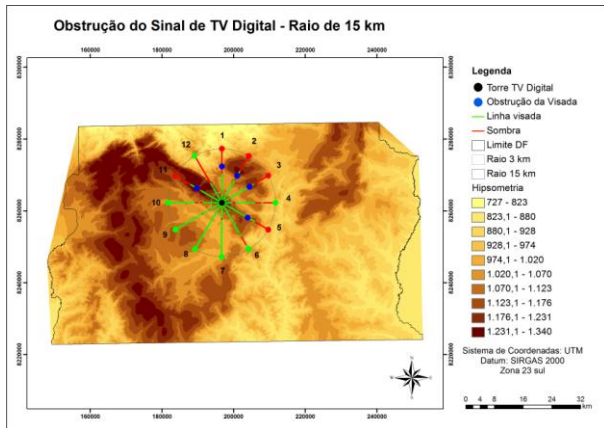
Fig.14 – Obstrução da linha de visada: contorno de 15km
