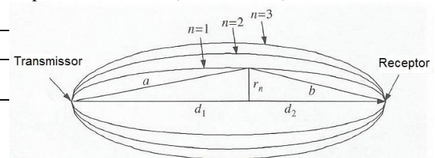
Fig.5 – Zonas de Fresnel. Fonte: SAUNDERS, 2007
