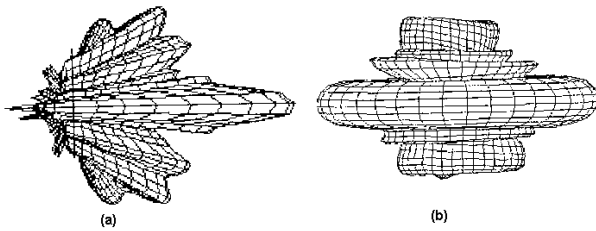
Fig.3 – Diagramas de irradiação vertical. (a) Antenas diretivas (ou setoriais). (b) Antenas Omnidirecionais.
