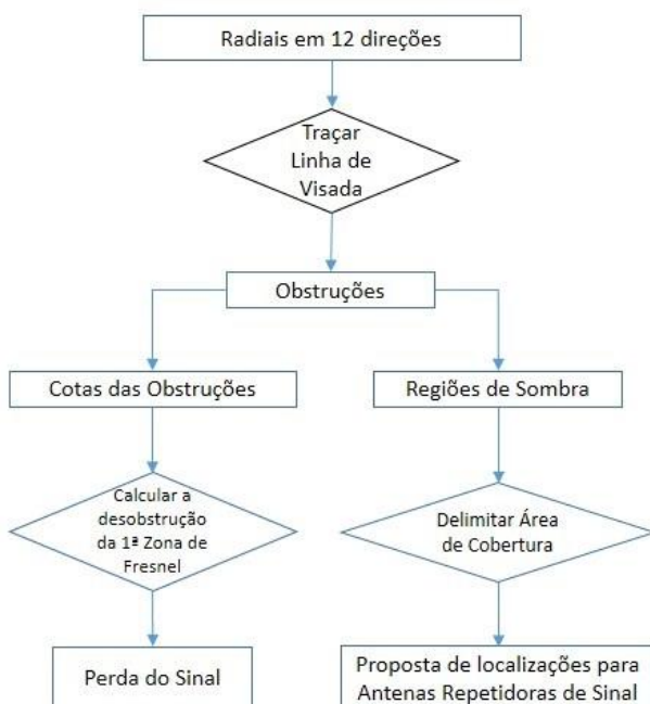
Fig.13 – Fluxograma da segunda etapa do procedimento
