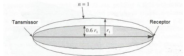
Fig.8 – Desobstrução da primeira Zona de Fresnel.
