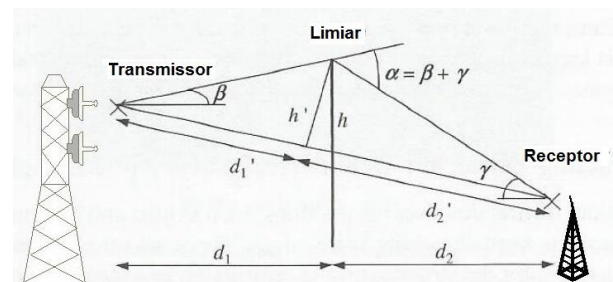
Fig.6 – Linha de Visada entre transmissor e receptor
