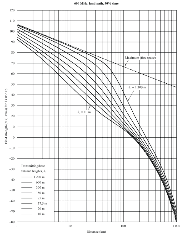
Fig.1 – Curvas de propagação do Modelo Okumura-Hata para frequência de 600MHz em percursos terrestres com 1kW de potência irradiada.
