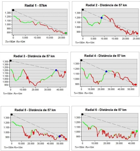
Fig. 19 - Contorno de 57km – Radiais de 1 a 6
