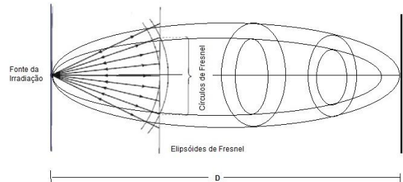
Fig. 4 – Elipsóides de Fresnel (fonte: Do Autor)
