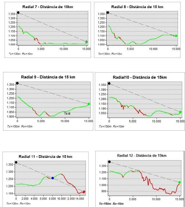
Fig.18– Contorno de 15km – Radiais de 7 a 12
