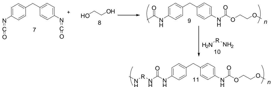
Esquema 2. Rota para síntese de copolímeros de Poliuretano-Poliuréia.
