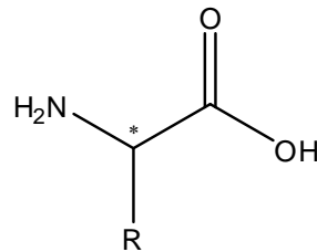
Figura 1. Estrutura básica de um aminoácido.
