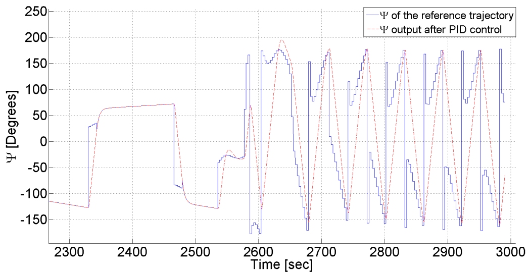
Figura 30 – Sinal de referência e o \psi atual sem vento.
