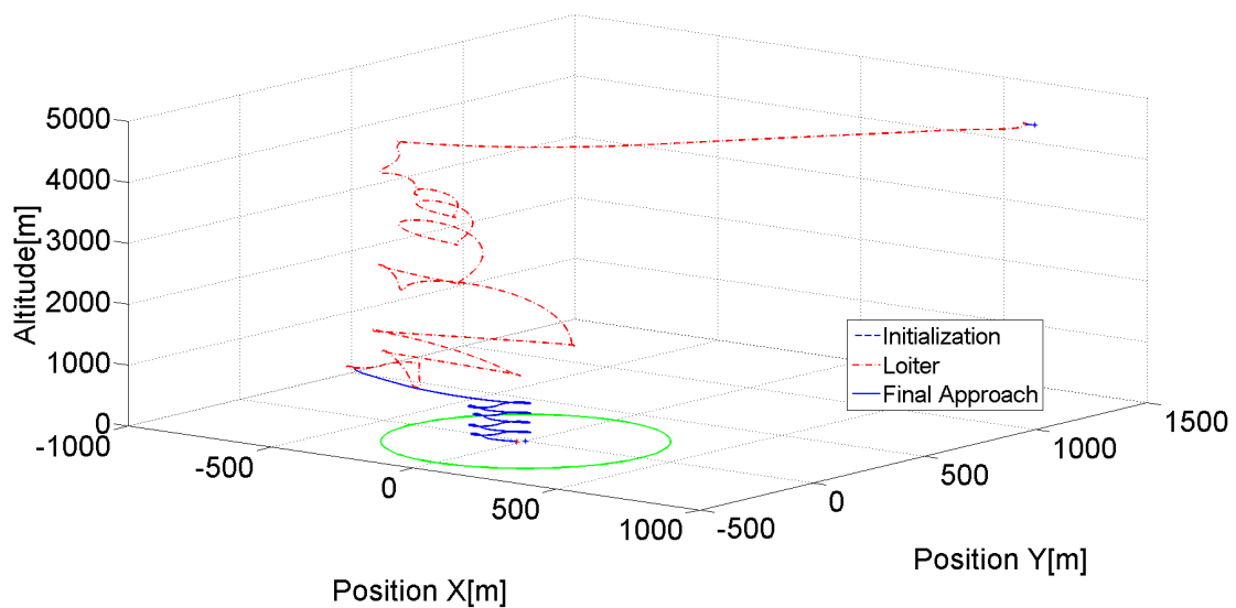
Figura 33 – Trajetória 3D com vento.
