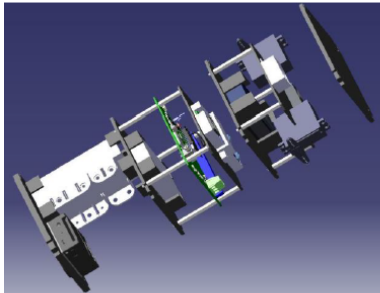
Figura 11 – Estrutura expandida do LAICAnSat-3.
