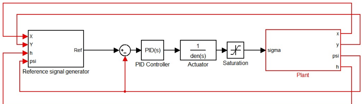
Figura 24 – Esquemático do sistema de controle.
