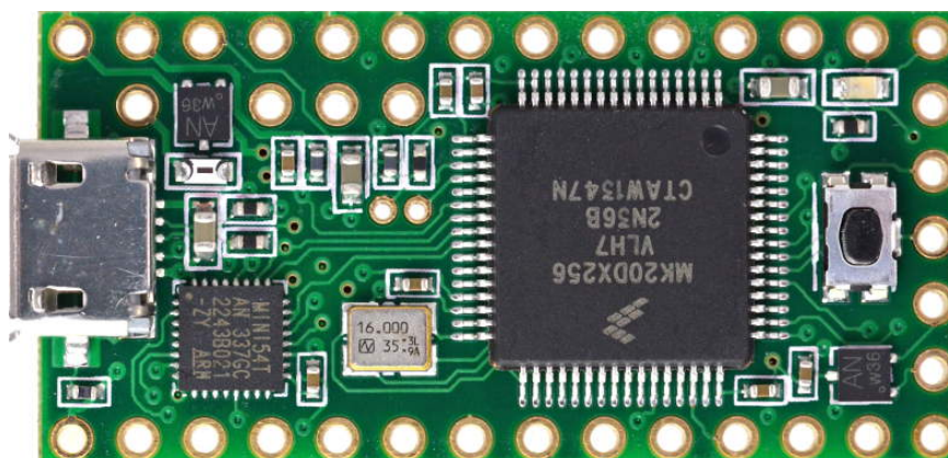
Figura 19 – Microcontrolador Teensy 3.1.
