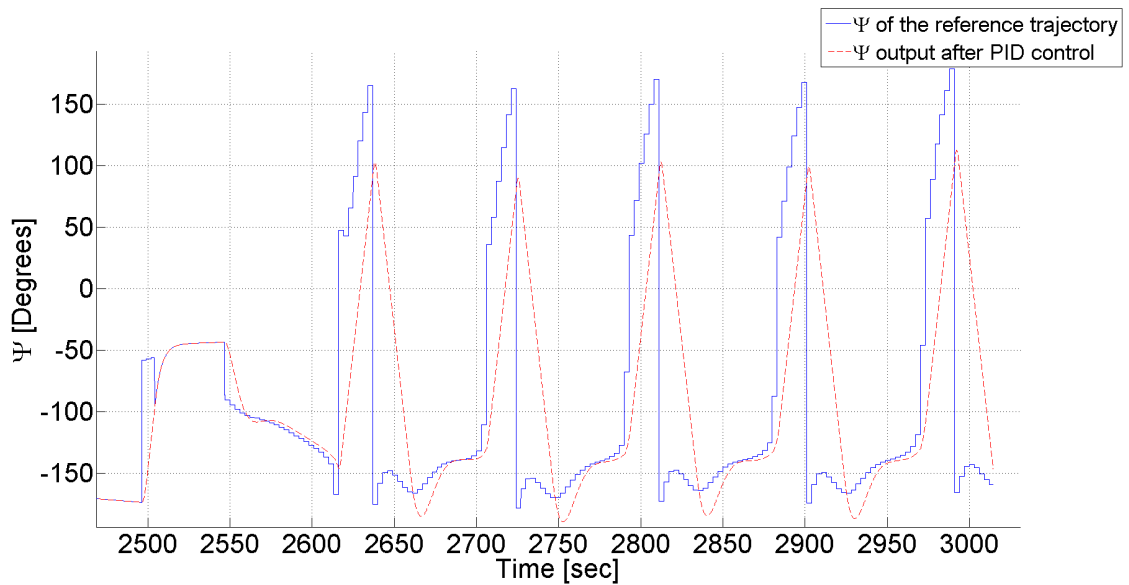
Figura 35 – Sinal de referência e o \psi atual com vento.
