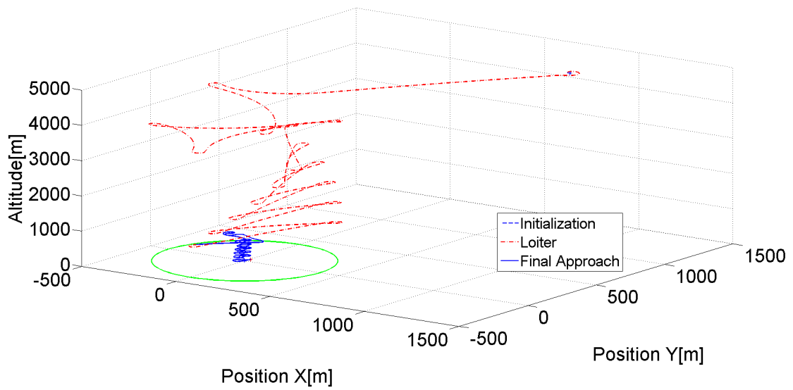
Figura 29 – Trajetória 3D sem vento.
