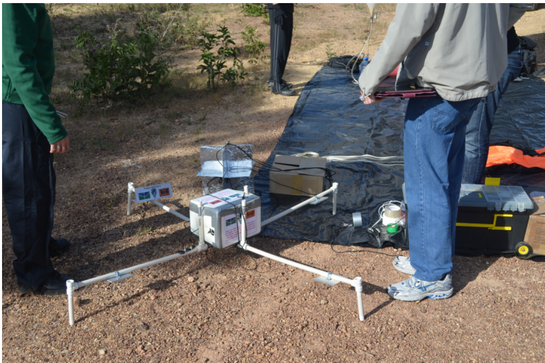
Figura 6 – Estrutura da carga útil montada antes do lançamento.
