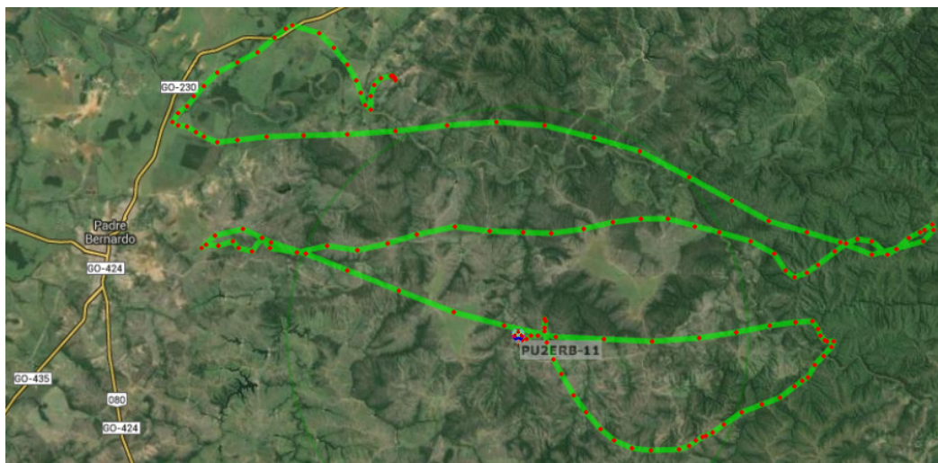
Figura 8 – Trajetória do Balloonsat dada pelo sistema APRS para o LAICAnSat-1.
