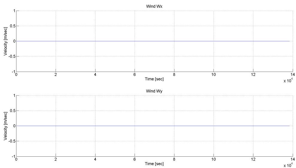
Figura 31 – Intensidade dos ventos.
