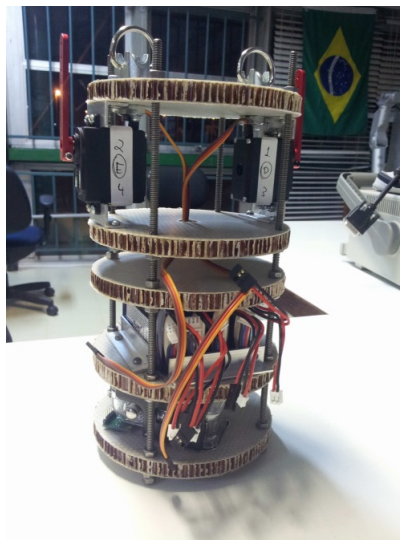
Figura 1 – Estrutura montada com a eletrônica do LAICAnSat-1 (NEHME et al., 2014).
