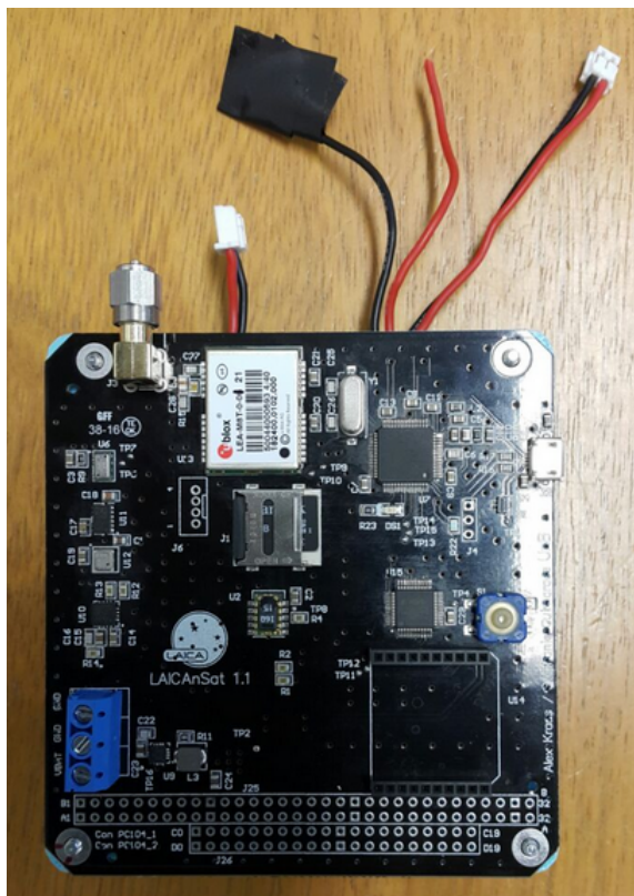
Figura 13 – Placa do computador de bordo do LAICAnSat-3.
