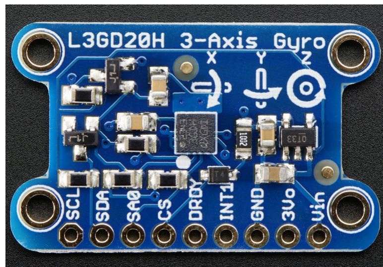
Figura 18 – Módulo L3GD20H.
