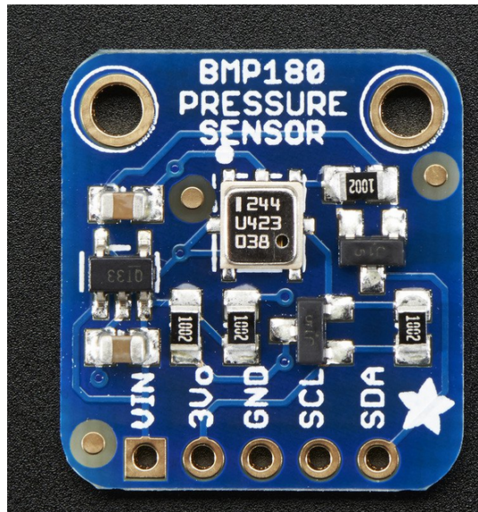
Figura 17 – Módulo BMP180.
