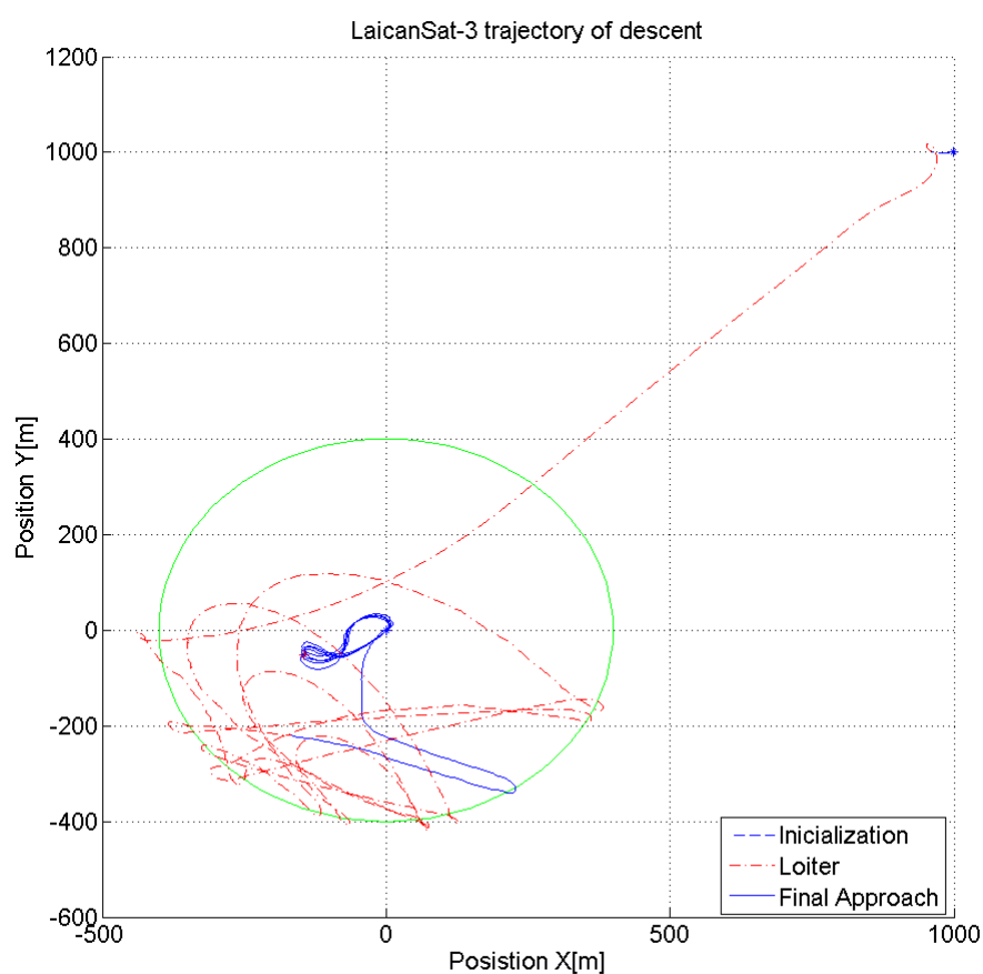
Figura 34 – Trajetória no plano XY com vento.
