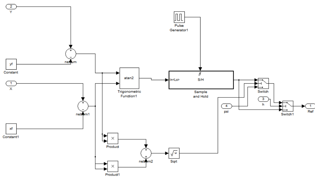
Figura 26 – Esquemático do bloco gerador do sinal de referência.
