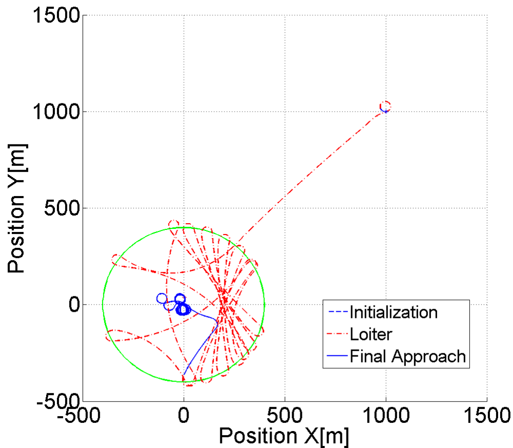
Figura 23 – As fases de descida do LAICAnSat-3 para o caso sem vento.
