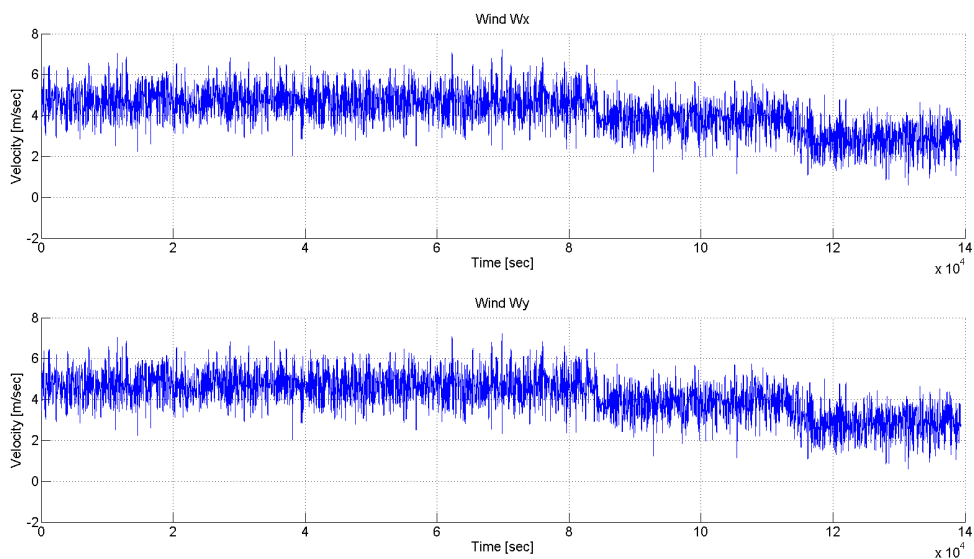
Figura 36 – Intensidade dos ventos
