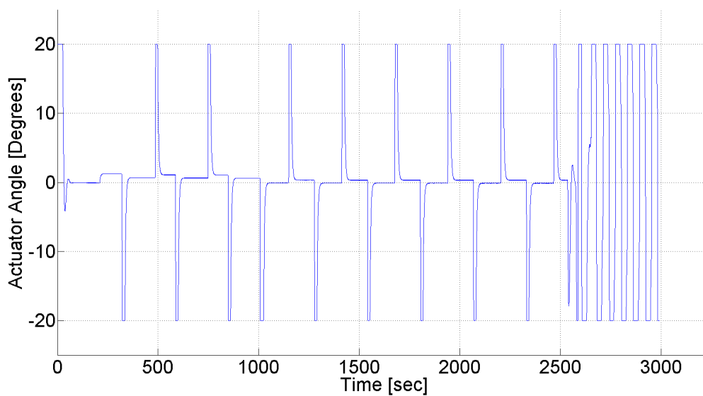
Figura 32 – Sinal gerado pelo atuador sem ventos.
