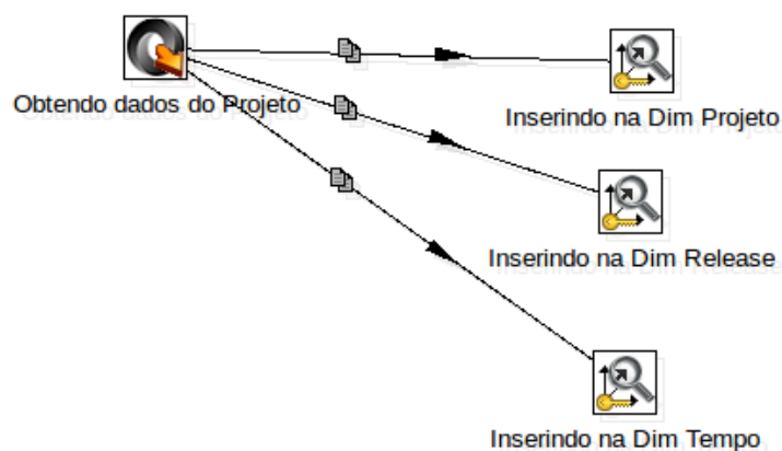
Figura 31 – Primeira Transforma o realizada no Kettle
