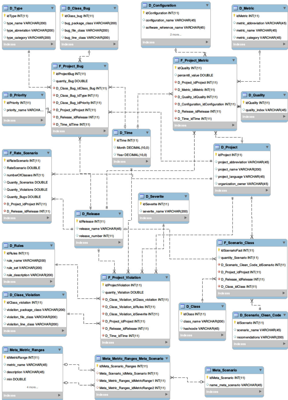
Figura 17 – Projeto físico do Data Warehouse finalizado.
