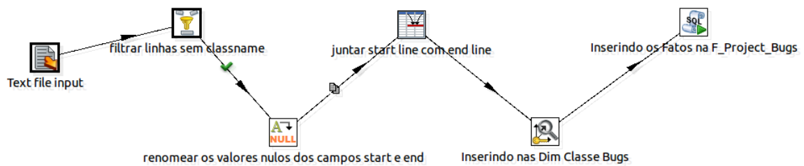
Figura 35 – Quinta Transformação realizada no Kettle
