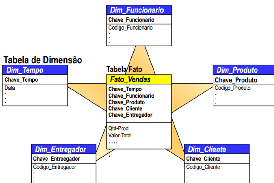
Figura 7 – Esquema estrela extraído de Times (2012)
