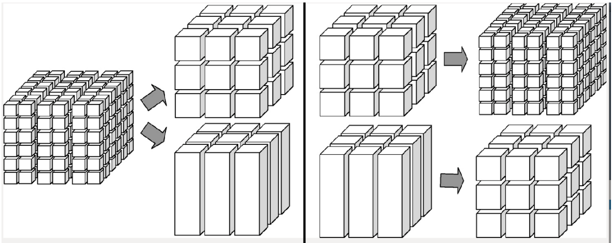
Figura 8 – Exemplo de operações Drill Down (direita) e Drill up (esquerda) extraídos de Golfarelli (2009)
