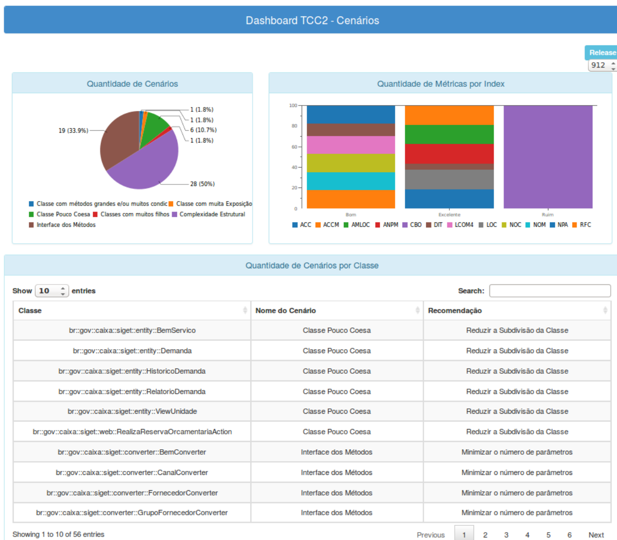
Figura 39 – Dashboard Cenários
