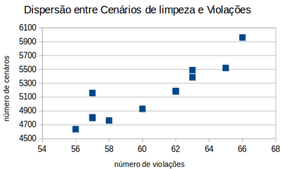
Figura 28 – Gráfico de Dispersão entre Cenários de Limpeza e Violações
